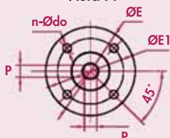
Vista A
